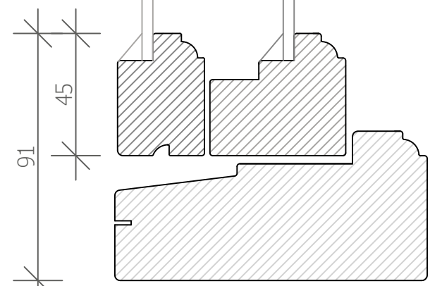
SIDOSTYCKE VERTIKALSNIITT
