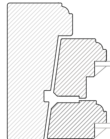
BOTTENSTYCKE HORIZONTALSNITT
