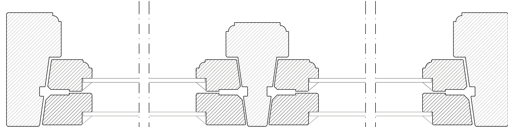
BOTTENSTYCKE HORIZONTALSNITT
