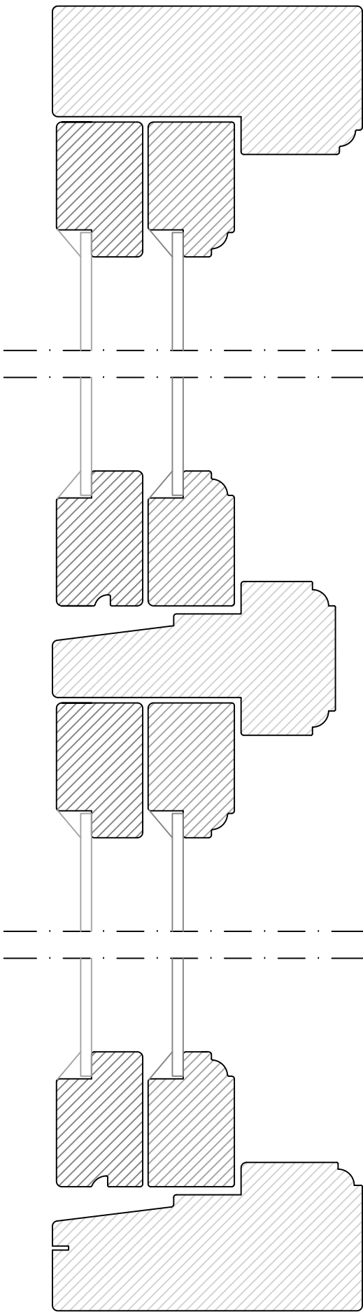
SIDOSTYCKE VERTIKALSNITT
