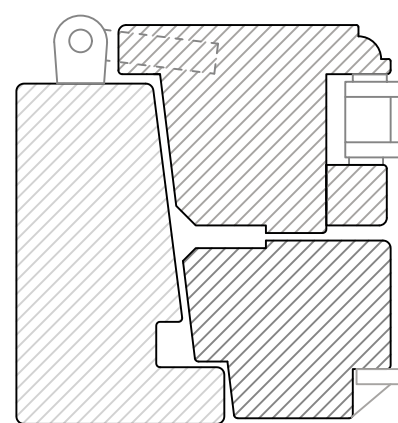
BOTTENSTYCKE HORIZONTALSNITT
