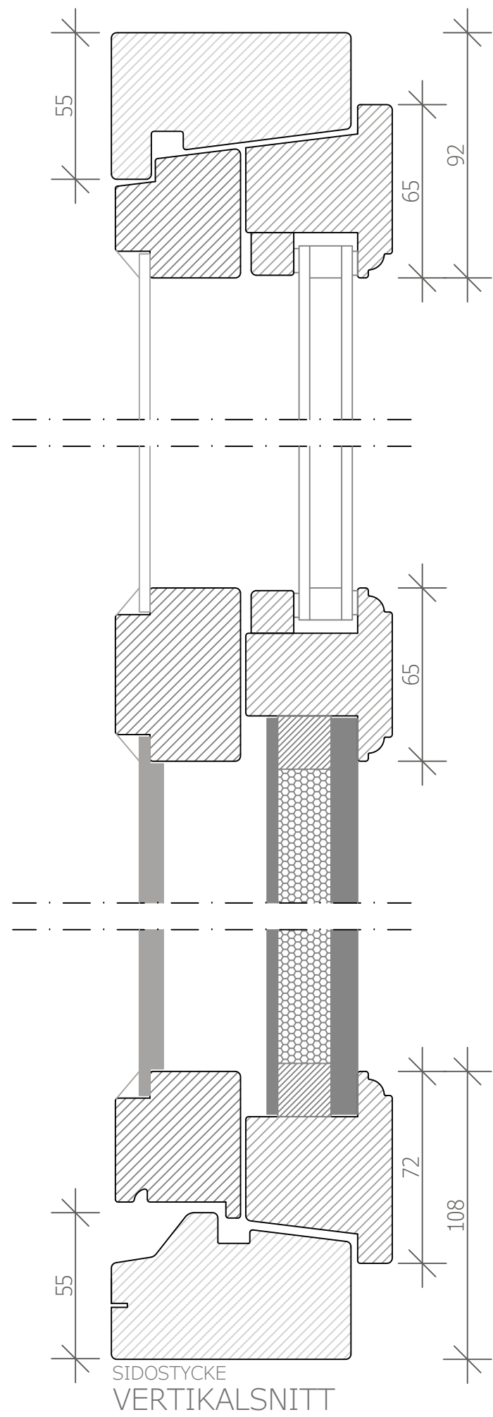
ALLMOGE PROFIL
