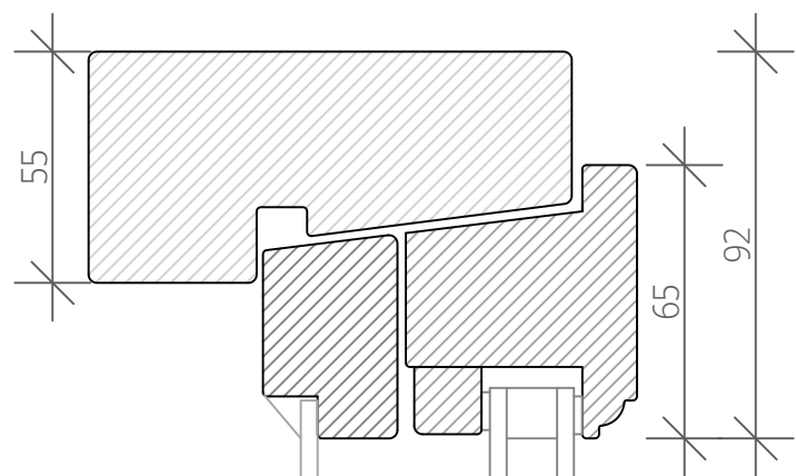
ALLMOGE PROFIL
