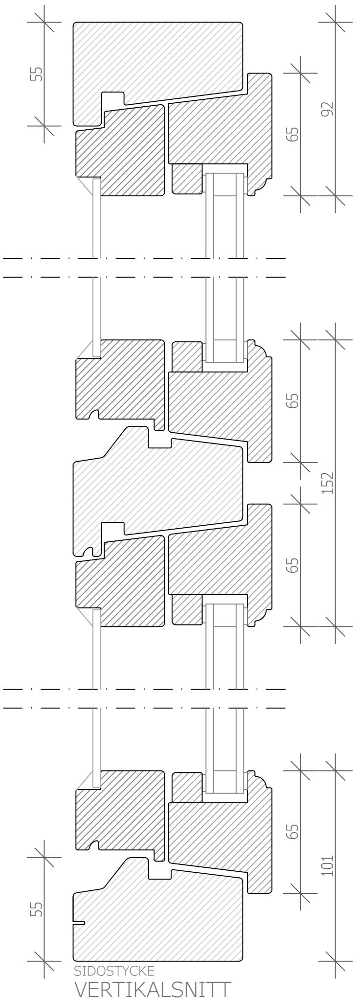
ALLMOGE PROFIL
