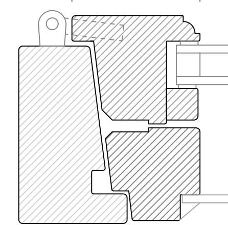
BOTTENSTYCKE HORIZONTALSNITT
