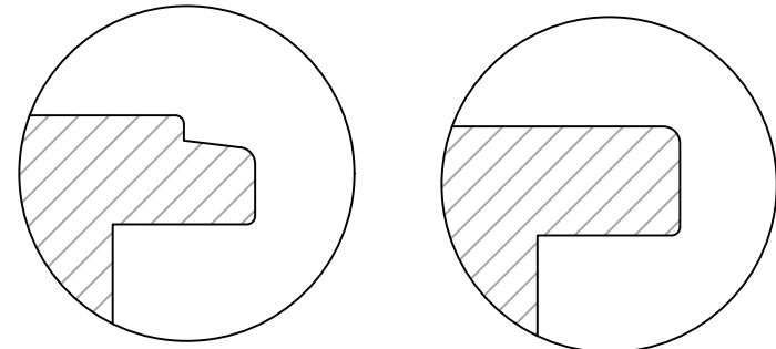
L-PROFIL
