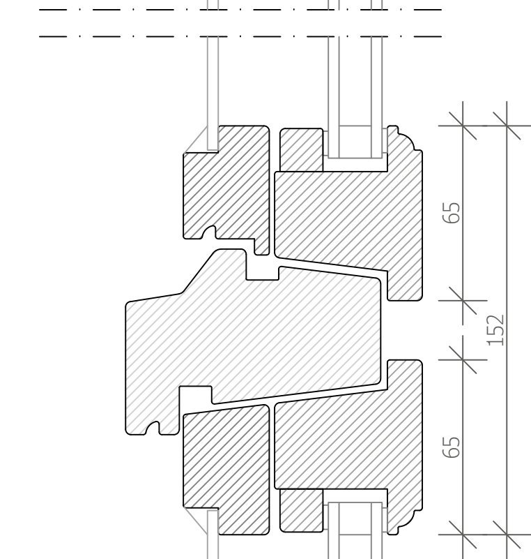
ALLMOGE PROFIL
