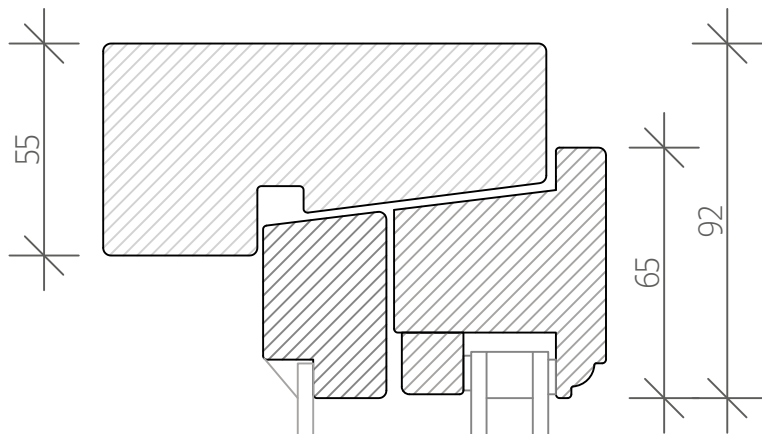
ALLMOGE PROFIL
