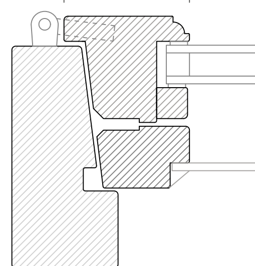
BOTTENSTYCKE HORIZONTALSNITT
