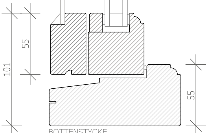
BOTTENSTYCKE VERTIKALSNITT
