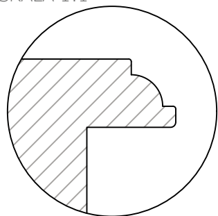
ALLMOGE PROFIL
