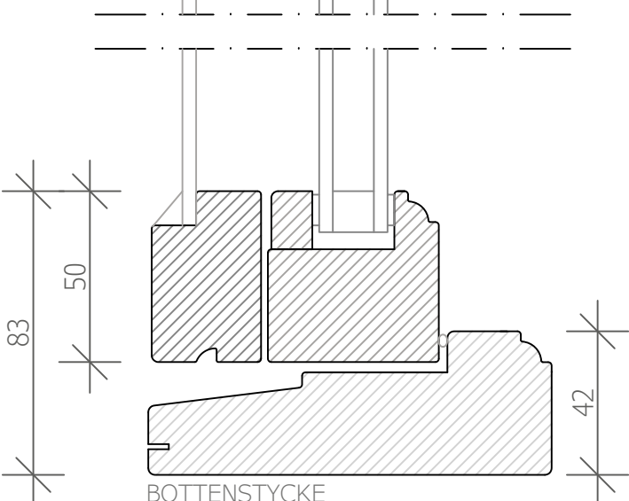
BOTTENSTYCKE VERTIKALSNIITT
