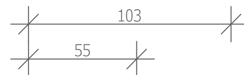
L-PROFIL
