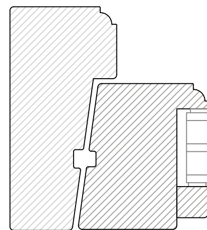
BOTTENSTYCKE HORIZONTALSNITT
