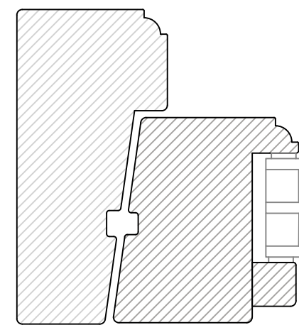
BOTTENSTYCKE HORIZONTALSNITT
